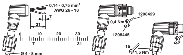
Dibujo funcional
